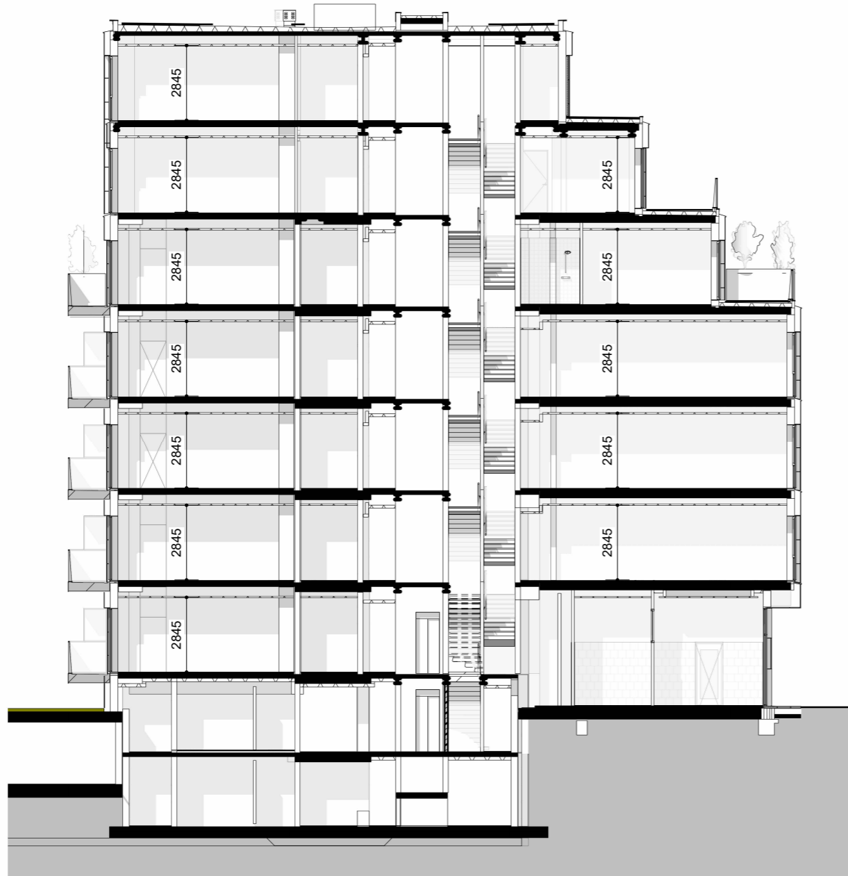
dwarsdoorsnede A-A 1 : 200
